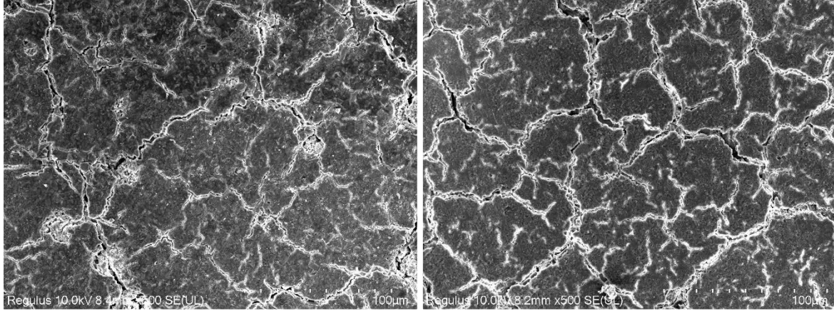
Şekil 2. (A) Equia Forte T0 SEM Görüntüsü (B) Sambucol ile yaşlandırılmış Equia Forte SEM Görüntüsü
