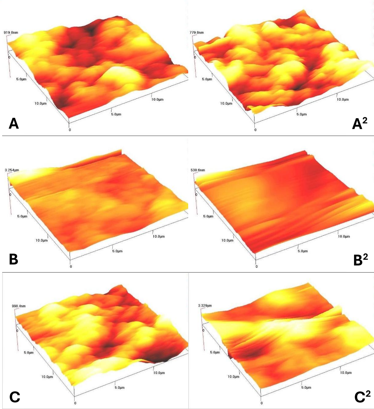
Şekil 1. Sırasıyla (A) Top – (A 2 ) Bottom T0, 919 ve 779 nm değerleri sahip rastgele seçilmiş AFM görüntüleri (B) Top – (B 2 ) Bottom T1_DS (3254 - 530 nm) AFM görüntüleri (C) Top – (C 2 ) Bottom T1_S (990 – 3300 nm) AFM görüntüleri
