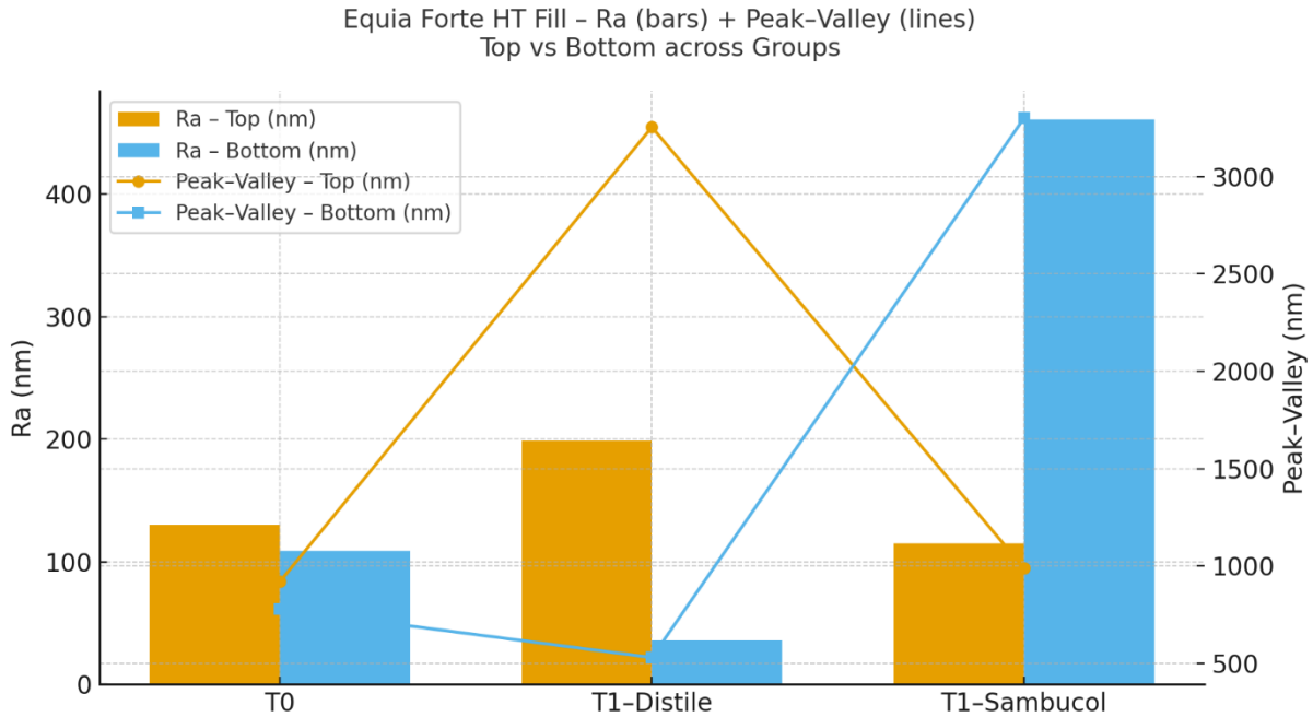
Şekil 3. Equia Forte HT Fil örneklerinde farklı yaşlandırma gruplarında üst ve alt yüzeylerin ortalama Ra ve Peak-Valley değerleri
