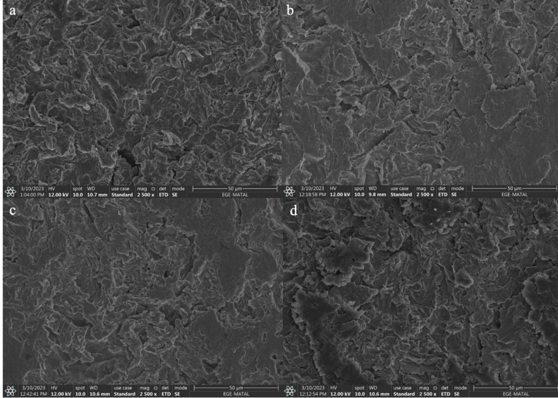
Şekil 1: Her bir gruba ait titanyum disklerin SEM görüntüleri
