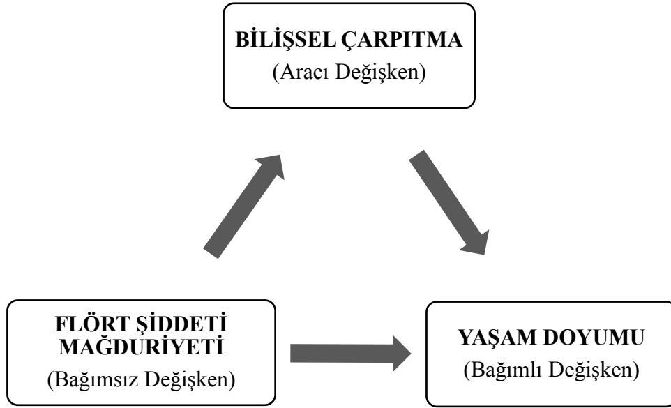
Şekil 3: Modelin Tanımlanması
