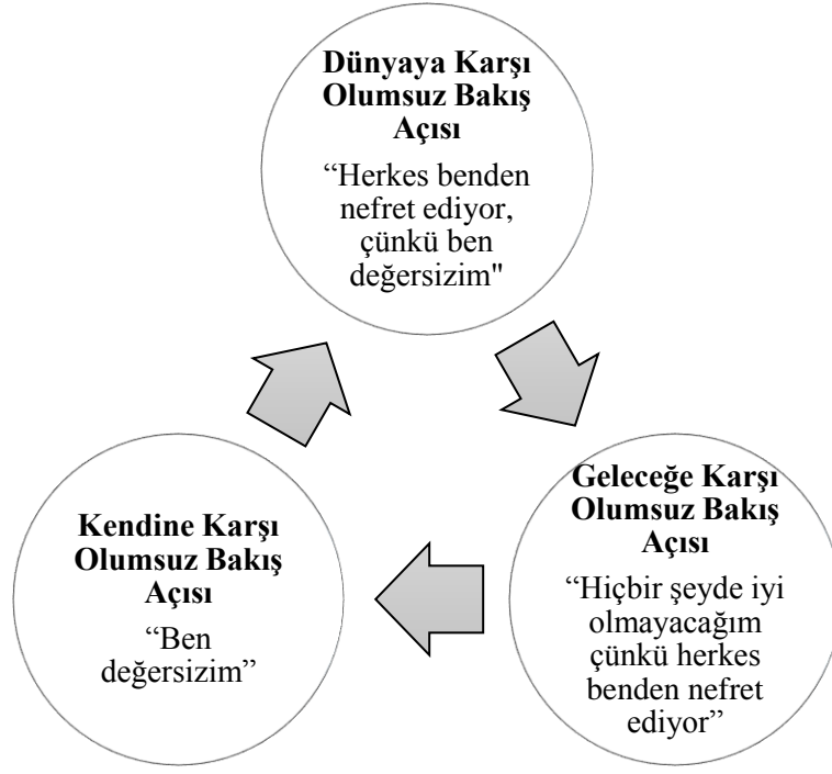
Şekil 2: Beck (1976) Negatif Temel İnançların Bilişsel Üçlüsü
